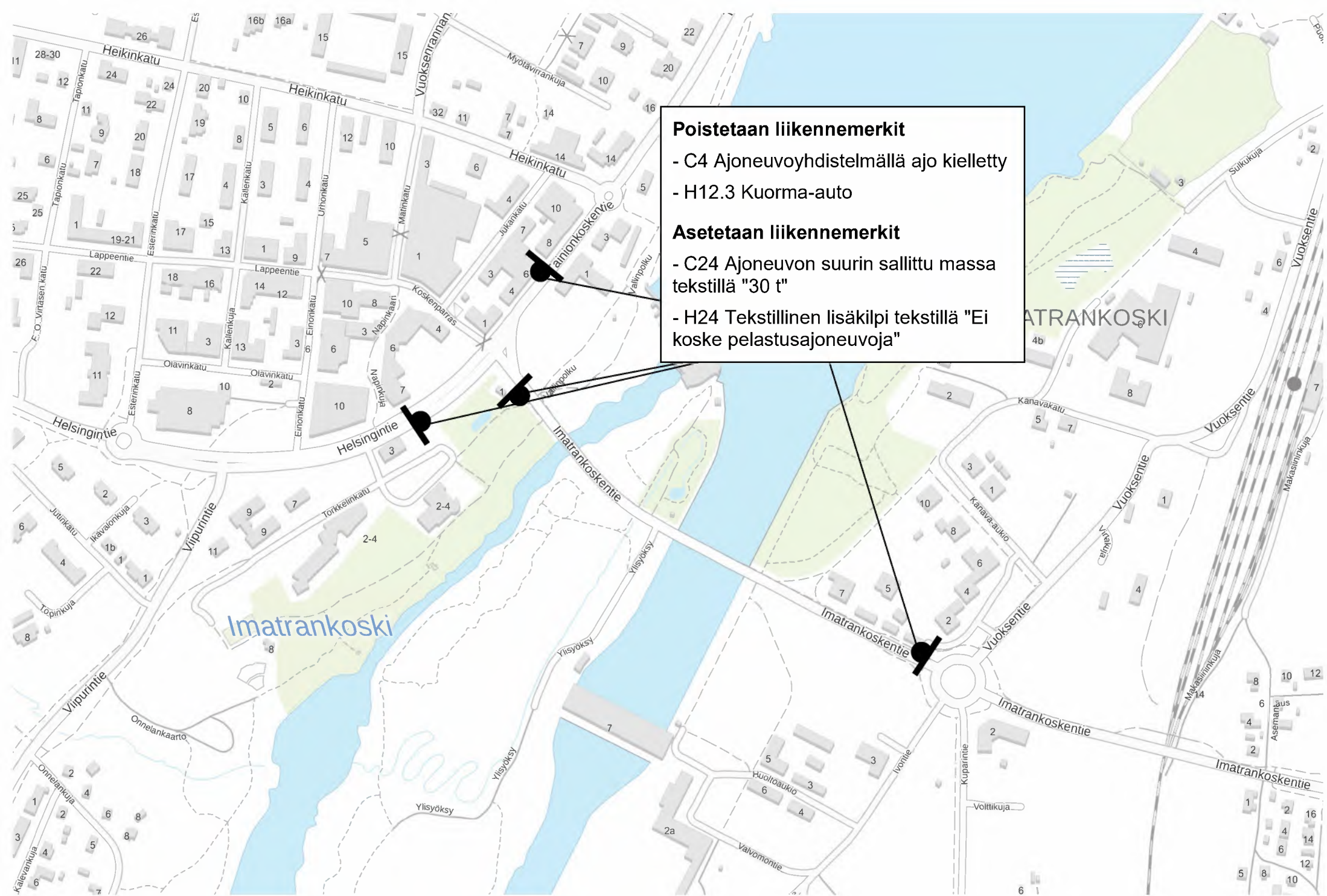
Liite 1, liikennemerkkisuunnitelma Imatrankosentie
