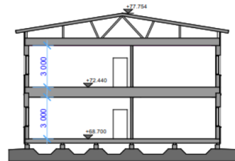
LEIKKAUS A-A 1:200
