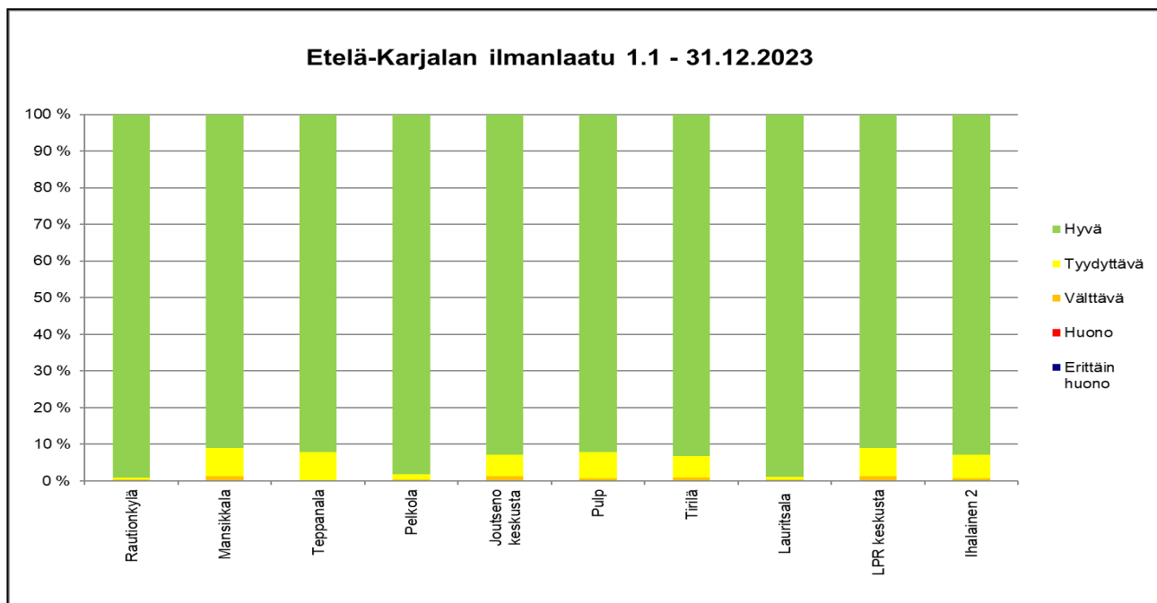
Kuva 58: Etelä-Karjalan ilmanlaatu eri mittauspisteillä tunti-indekseillä kuvattuna vuonna 2023
