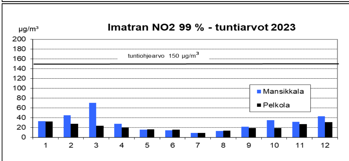
Kuvat 21: Imatran mittauspisteiden NO 2 - kuukausikeskiarvot ja NO 2 - kuukausien 99 % - tuntikeskiarvot (µg/m 3 ) vuonna 2023
