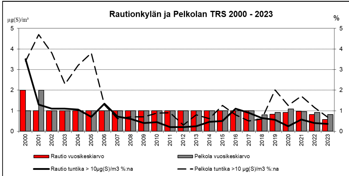
Kuva 14a: Rautionkylän ja Pelkolan TRS-yhdisteiden vuosikeskiarvot ja tuntikeskiarvon 10 µg(S)/m 3 ylittäneiden tuntikeskiarvojen osuudet vuosina 2000–2023
