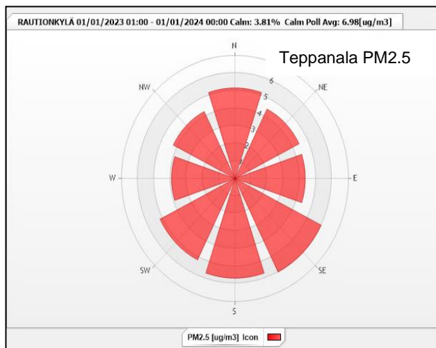
Kuva 28: Imatran Teppanalan mittauspisteen PM2,5:n pitoisuuksien tuulensuuntajakaumat vuonna 2023. Rautionkylän sääaseman tuulensuunta, tuulennopeus \geq 0,3 m/s.
