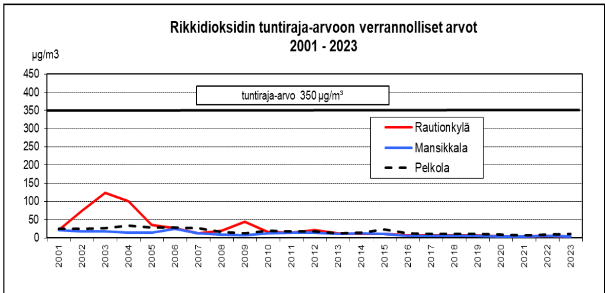
Kuva 19: Imatran Rautionkylän, Mansikkalan ja Pelkolan mittauspisteiden rikkidioksidin tuntiraja-arvoon verrannolliset tunnusluvut (25. suurimmat arvot) vuosina 2001 – 2023
