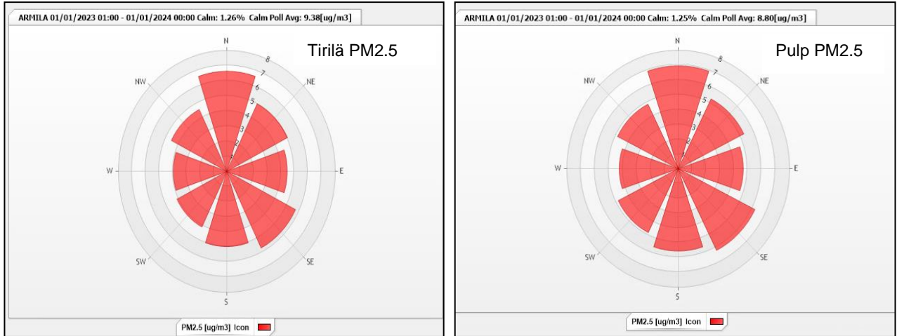
Kuva 54: Tirilän ja Pulpin PM2,5 - tuntikeskiarvojen tuulensuuntajakaumat sektoreittain vuonna 2023. Armilan tuulensuunta, tuulennopeus \geq 0,3 m/s.
