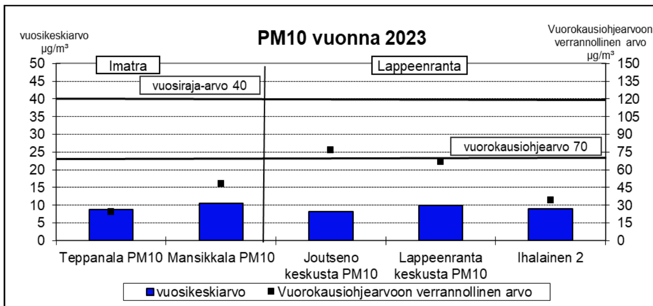
Kuva 63: PM10:n vuosikeskiarvot ja vuorokausiohjearvoon verrannolliset arvot vuonna 2023 Imatralla ja Lappeenrannassa
