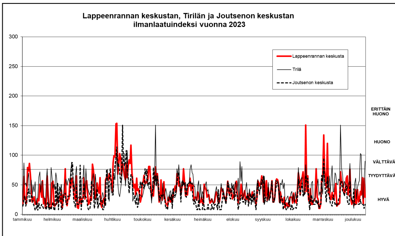
Kuva 30: Ilmanlaatu ilmanlaatuindeksin mukaan Lappeenrannan keskustassa, Tirilässä ja Joutsenon keskustassa vuonna 2023
