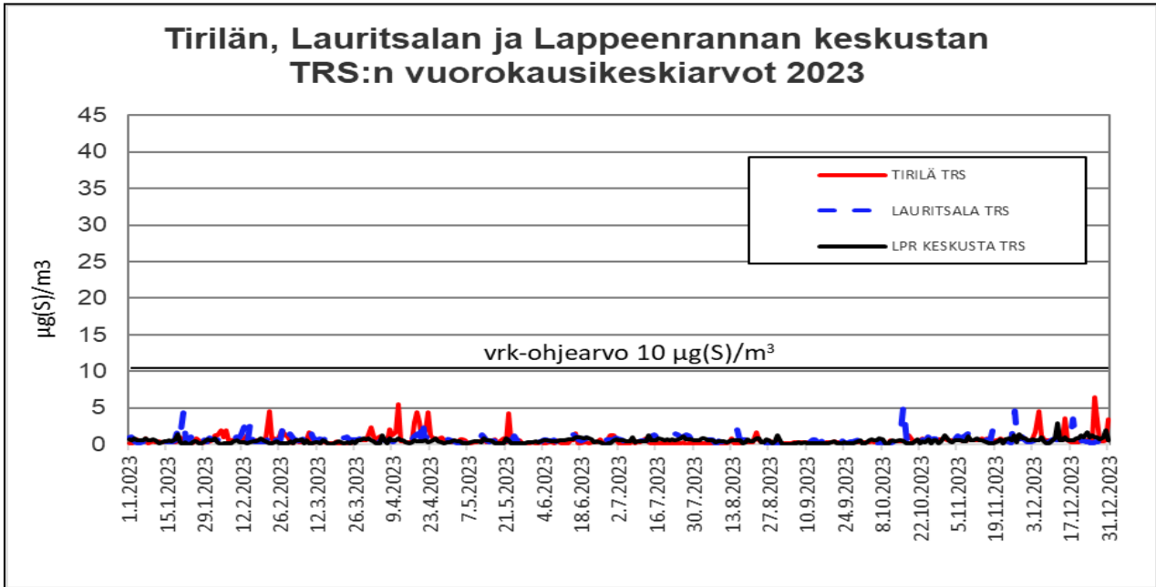
Kuva 31: Tirilän, Lauritsalan ja Lappeenrannan keskustan mittauspisteiden TRS - yhdisteiden vuorokausikeskiarvot ( \mu\text{g(S)}/\text{m}^3 ) vuonna 2023
