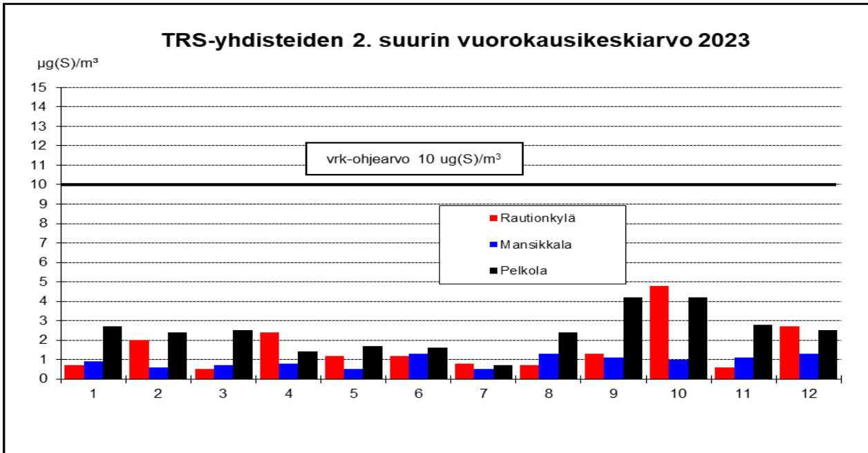
Kuva 13: Imatran mittauspisteiden TRS-yhdisteiden suurimmat tuntikeskiarvot ( \mu\text{g(S)}/\text{m}^3 ) ja TRS-yhdisteiden kuukausien toiseksi suurimmat vuorokausikeskiarvot ( \mu\text{g(S)}/\text{m}^3 ) vuonna 2023
