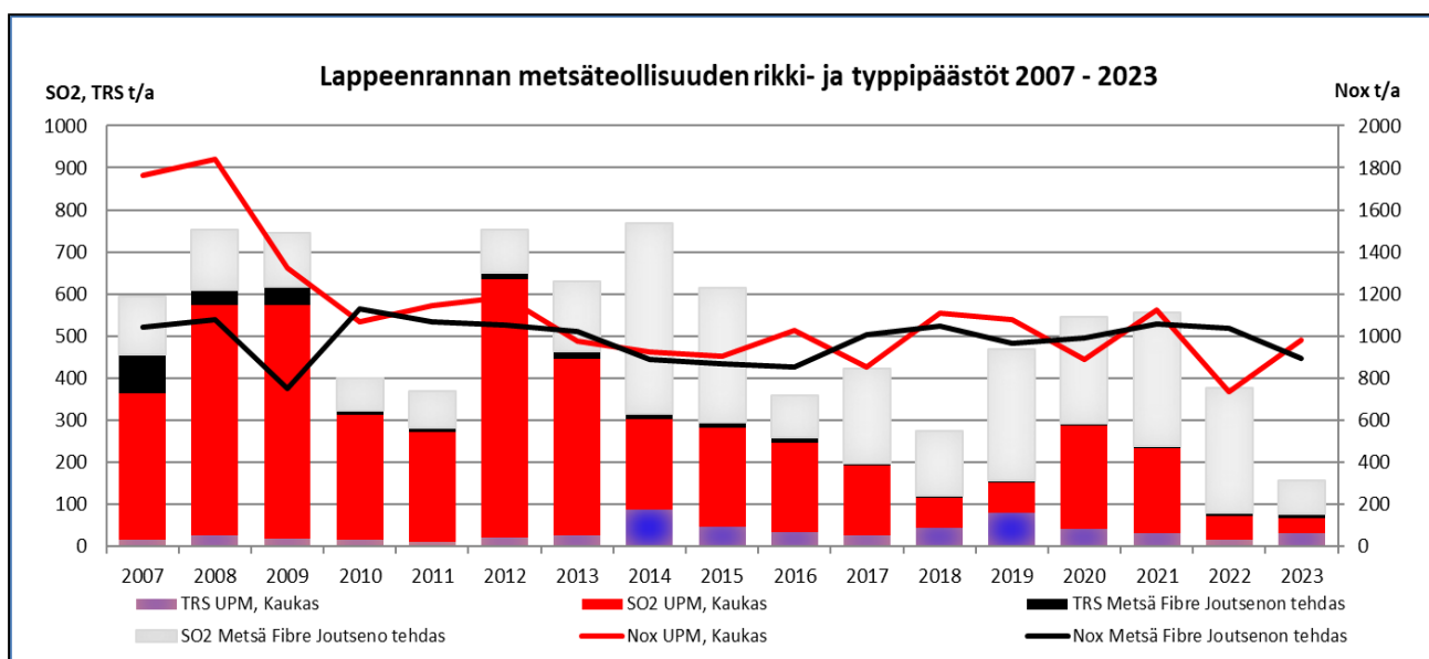
Kuva 4: Lappeenrannan tehtaiden TRS-, SO 2 - ja NO x - päästöt (t/a) vuosina 2007 - 2023 (Pylväsdiagrammien asteikko vasemmalla ja viivadiagrammien asteikko oikealla)
