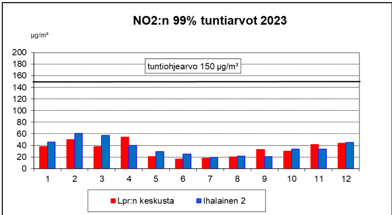
Kuva 44: Lappeenrannan mittauspisteiden NO 2 - kuukausikeskiarvot ja NO 2 - tuntiohjearvoon (99 % - tuntiarvot) verrattavat tunnusluvut vuonna 2023 (µg/m 3 )
