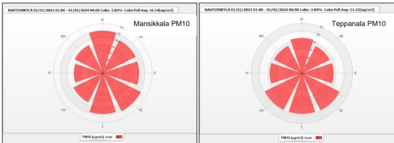
Kuva 27: Imatran Mansikkalan ja Teppanalan mittauspisteiden PM10:n pitoisuuksien tuulensuuntajakaumat vuonna 2023. Rautionkylän sääaseman tuulensuunta, tuulennopeus \geq 0,3 m/s.
