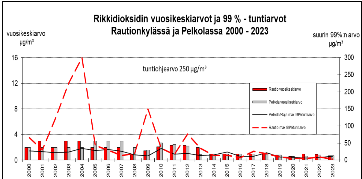
Kuva 18: Imatran Rautionkylän ja Pelkolan rikkidioksidin vuosikeskiarvot ja suurimmat 99 % tunti-arvot vuosina 2000 – 2023
