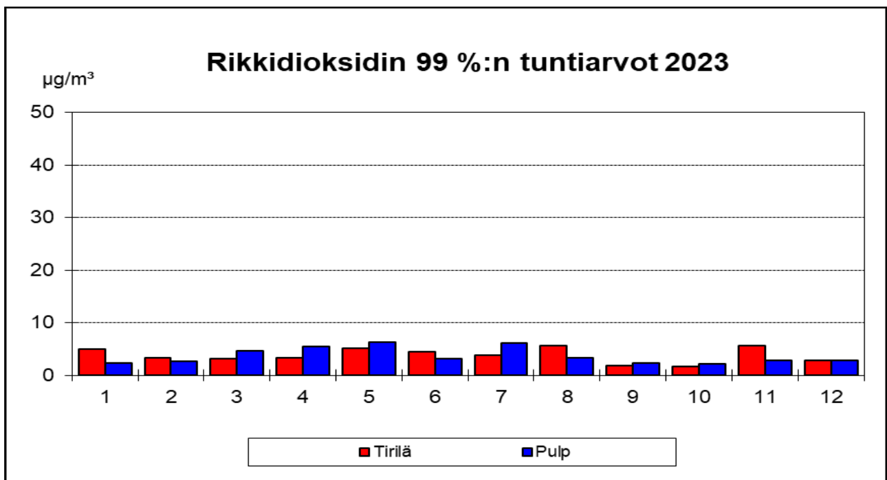
Kuva 38: Lappeenrannan mittauspisteiden rikkidioksidin kuukausikeskiarvot ja 99 % - tuntikeskiarvot vuonna 2023 (µg/m 3 ).
