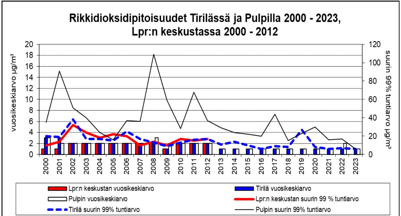
Kuva 41: Tirilän ja Pulpin mittauspisteiden rikkidioksidin vuosikeskiarvot ja suurimmat 99 % -tuntikeskiarvot vuosina 2000 – 2023, sekä Lappeenrannan keskustan rikkidioksidin vuosikeskiarvot ja suurimmat 99 % -tuntikeskiarvot vuosina 2000 – 2012
