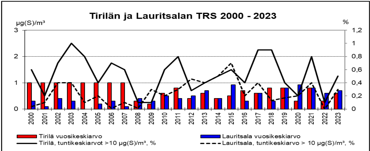
Kuva 35: Tirilän ja Lauritsalan mittauspisteiden TRS - yhdisteiden vuosikeskiarvot ja tuntikeskiarvon 10 \mu\text{g(S)}/\text{m}^3 ylitysosuudet (%) vuosina 2000 – 2023
