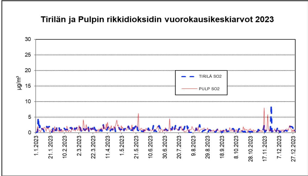
Kuva 39: Tirilän ja Pulpin mittauspisteiden rikkidioksidin vuorokausikeskiarvot vuonna 2023 ( \mu\text{g}/\text{m}^3 ).
