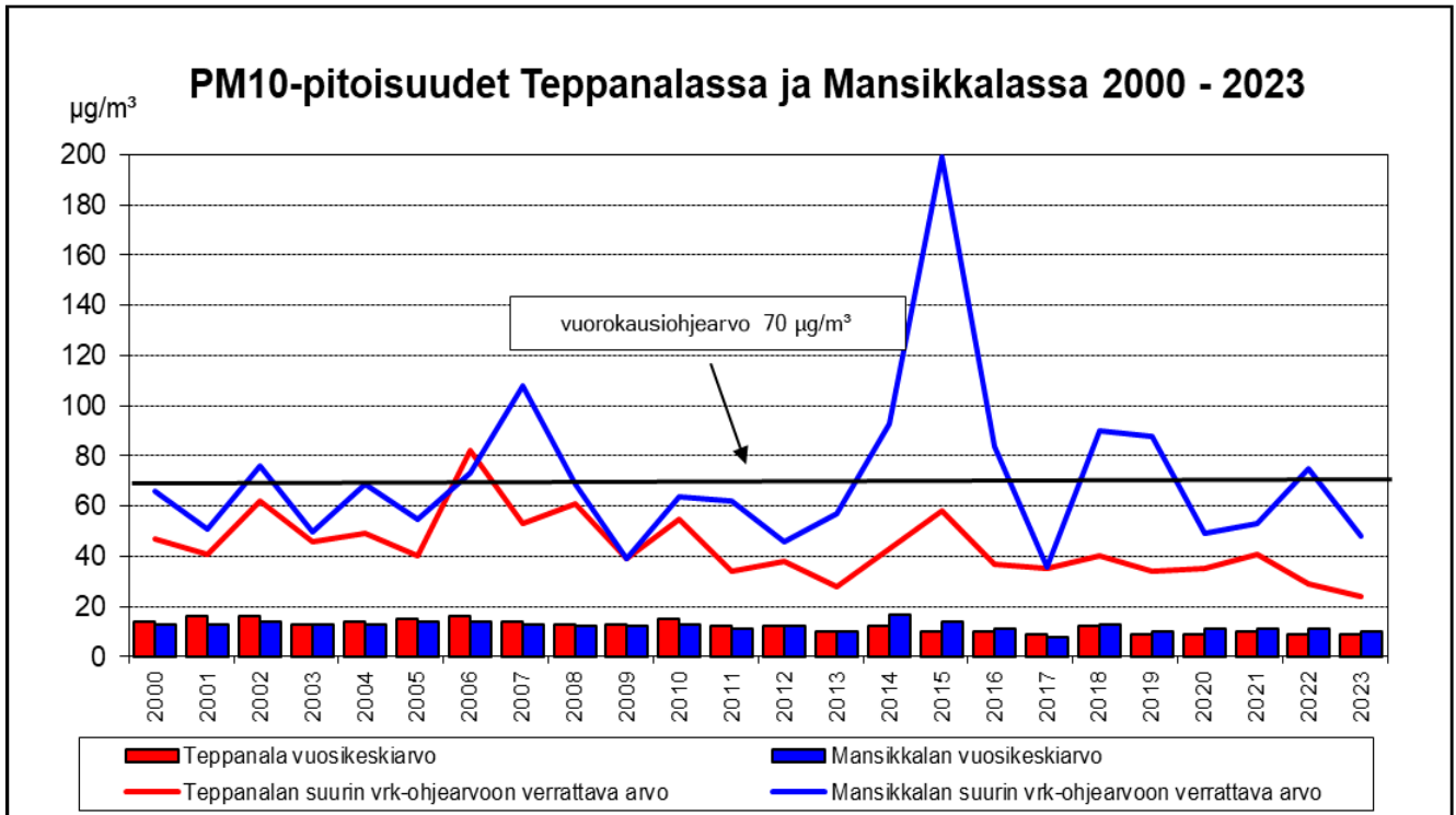
Kuva 29: Imatran Teppanalan ja Mansikkalan mittauspisteiden PM10 - vuosikeskiarvot ja suurimmat vuorokausiohjearvoon verrattavat arvot vuosina 2000 – 2023
