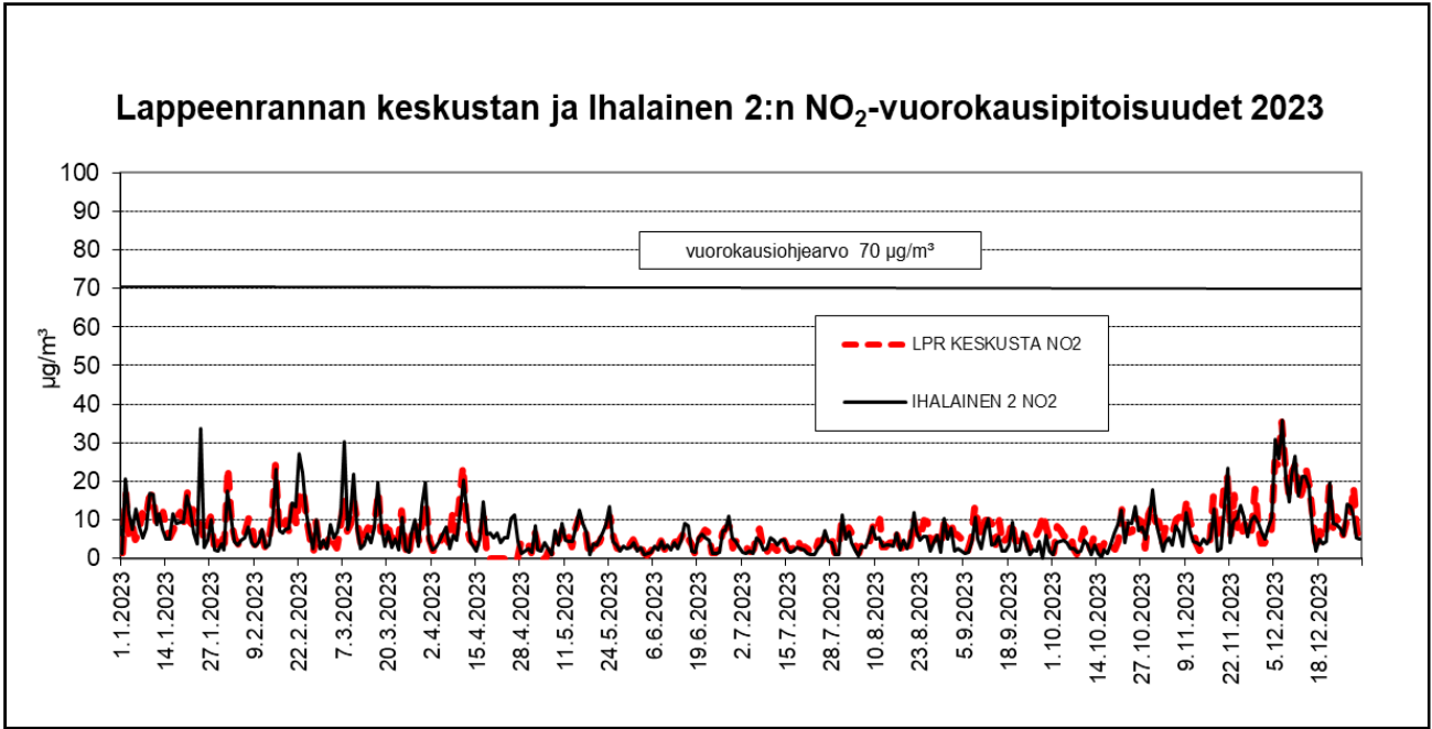
Kuva 42: Lappeenrannan keskustan ja Ihalainen 2:n NO 2 - vuorokausikeskiarvot vuonna 2023 (µg/m 3 ).
