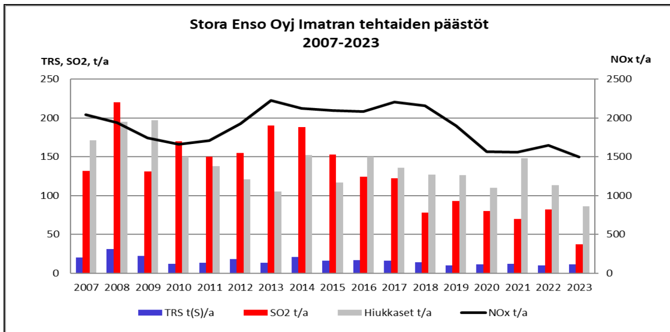
Kuva 2: Stora Enso Oyj Imatran tehtaiden ilmapäästöt vuosina 2007 - 2023 (Pylväsdiagrammien asteikko vasemmalla ja viivadiagrammin asteikko oikealla)
