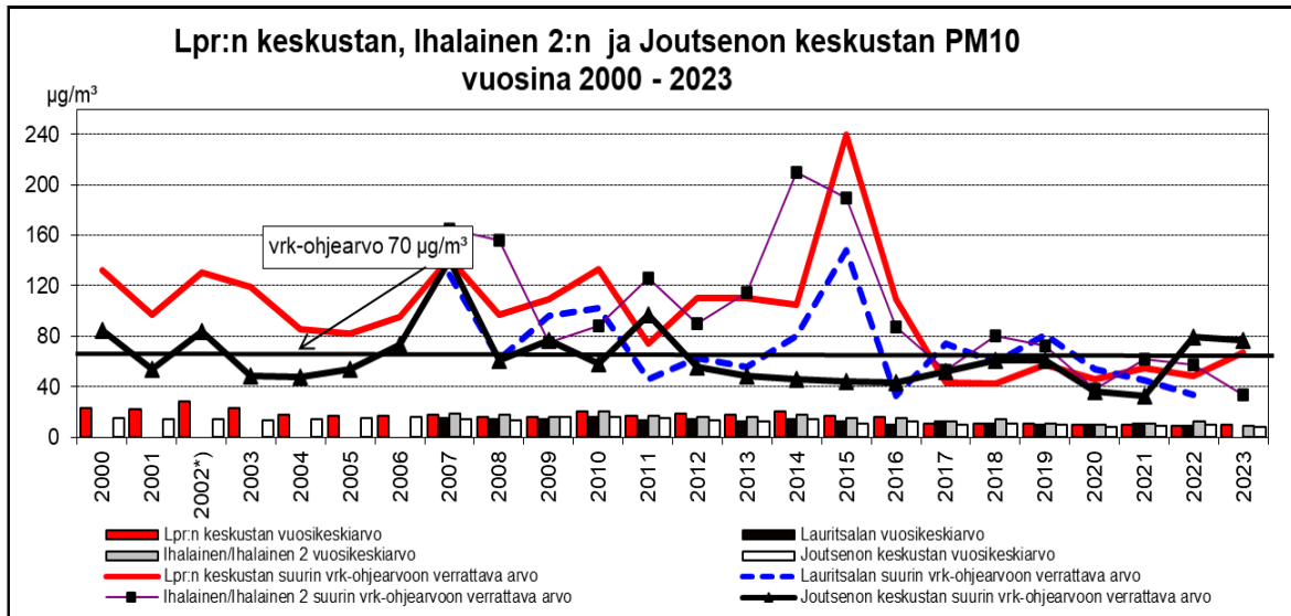
Kuva 50: Lappeenrannan hiukkasmittauspisteiden PM10 - vuosikeskiarvot ja suurimmat kuukausien toiseksi suurimmista vuorokausikeskiarvoista vuosina 2000 – 2023, Ihalaisen mittauspisteiden sijainti muuttunut 30.5.2022 ja nimetty Ihalainen 2:ksi
