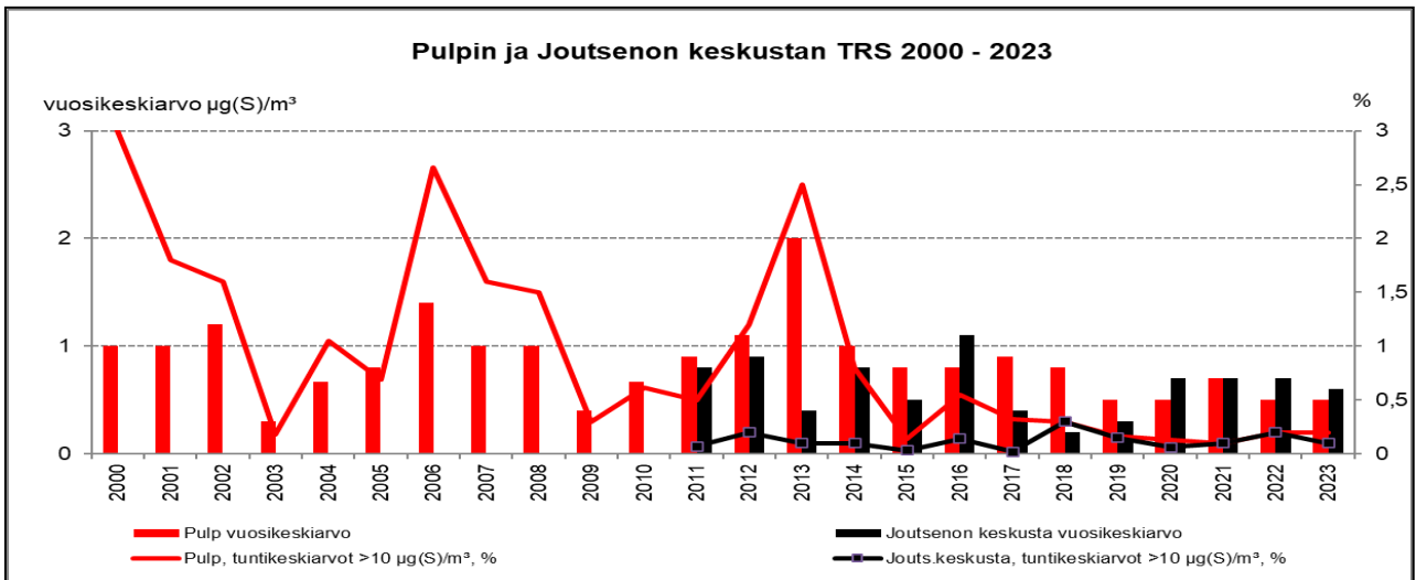
Kuva 36: Pulpin ja Joutsenon keskustan mittauspisteiden TRS - yhdisteiden vuosikeskiarvot ja tuntikeskiarvon 10 \mu\text{g(S)}/\text{m}^3 ylitysosuudet (%) vuosina 2000 – 2023
