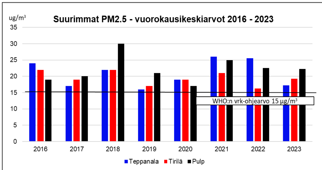
Kuva 65: PM 2,5 :n suurimmat vuorokausikeskiarvot vuosina 2016 - 2023 Imatralla ja Lappeenrannassa
