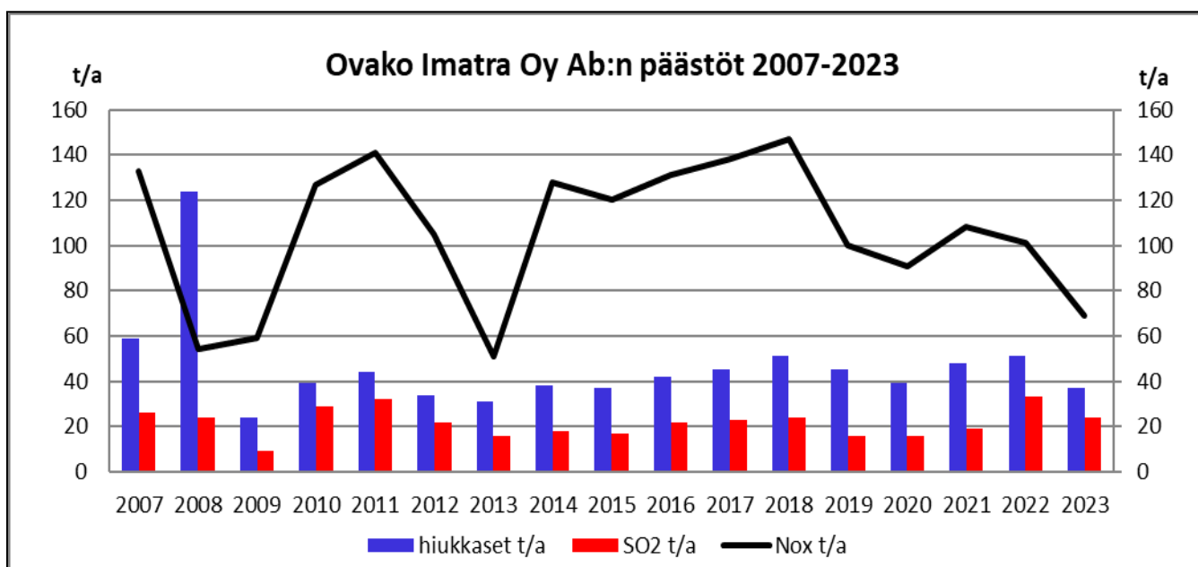
Kuva 3: Ovako Imatra Oy Ab:n ilmapäästöt (t/a) vuosina 2007 -2023
