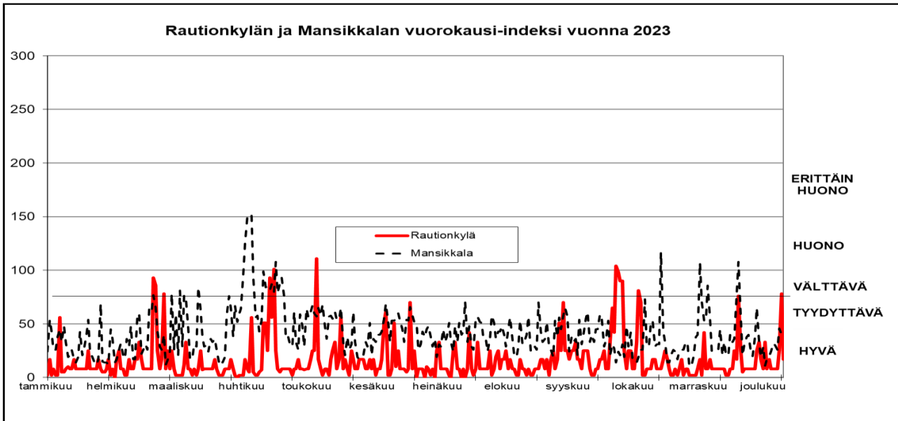
Kuva 10: Rautionkylän ja Mansikkalan ilmanlaatu vuorokausi-indeksillä kuvattuna vuonna 2023
