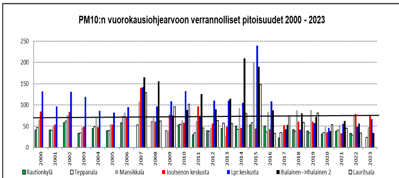
Kuva 64: PM10:n suurimmat kuukauden toiseksi suurimmista vuorokausikeskiarvoista vuosina 2000 – 2023 (Ihalainen vaihtui Ihalainen 2:ksi kesäkuussa 2022)
