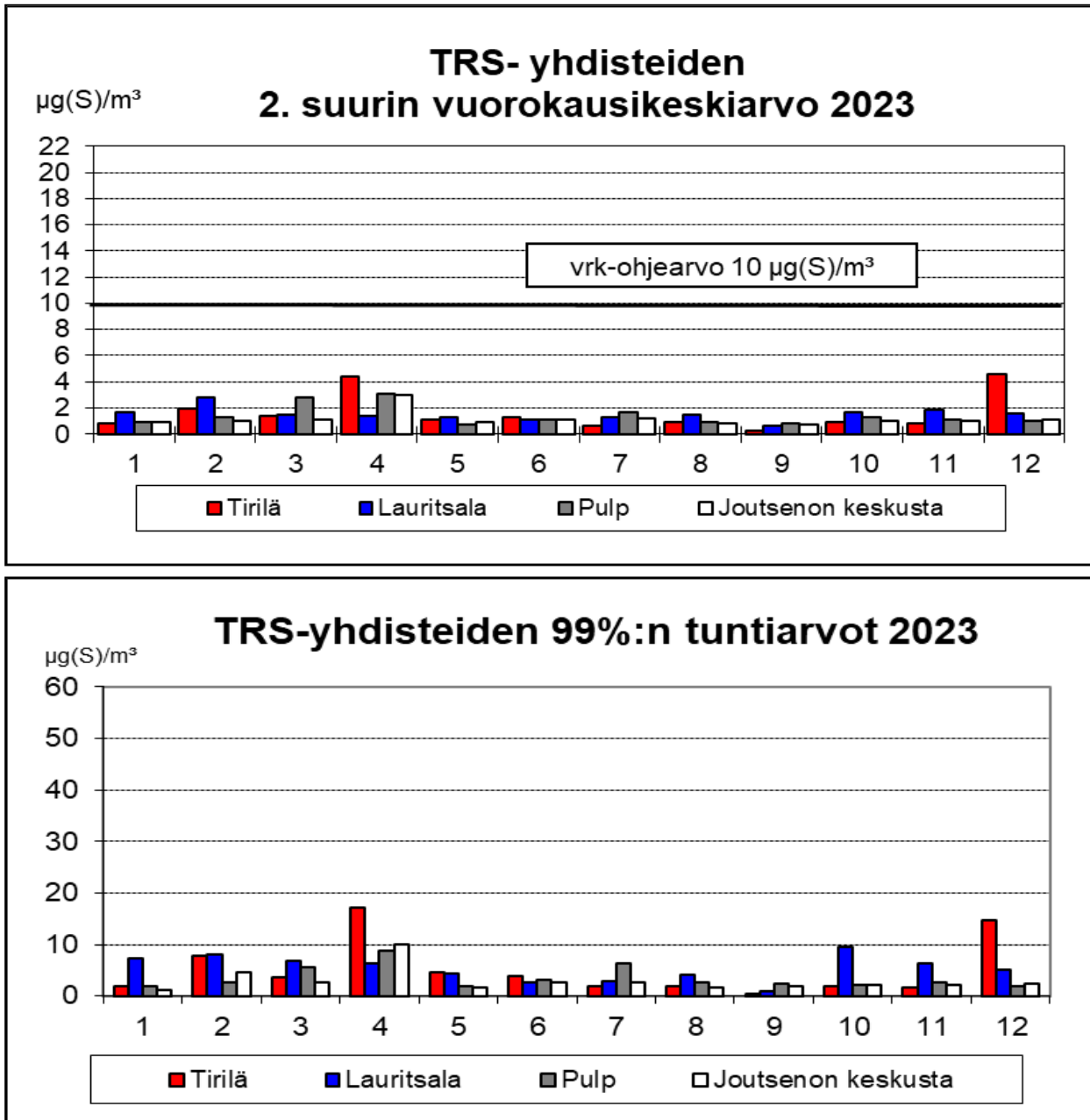
Kuva 34: Lappeenrannan mittauspisteiden TRS-yhdisteiden toiseksi suurimmat vuorokausikeskiarvot ja 99 % - tuntiarvot vuonna 2023
