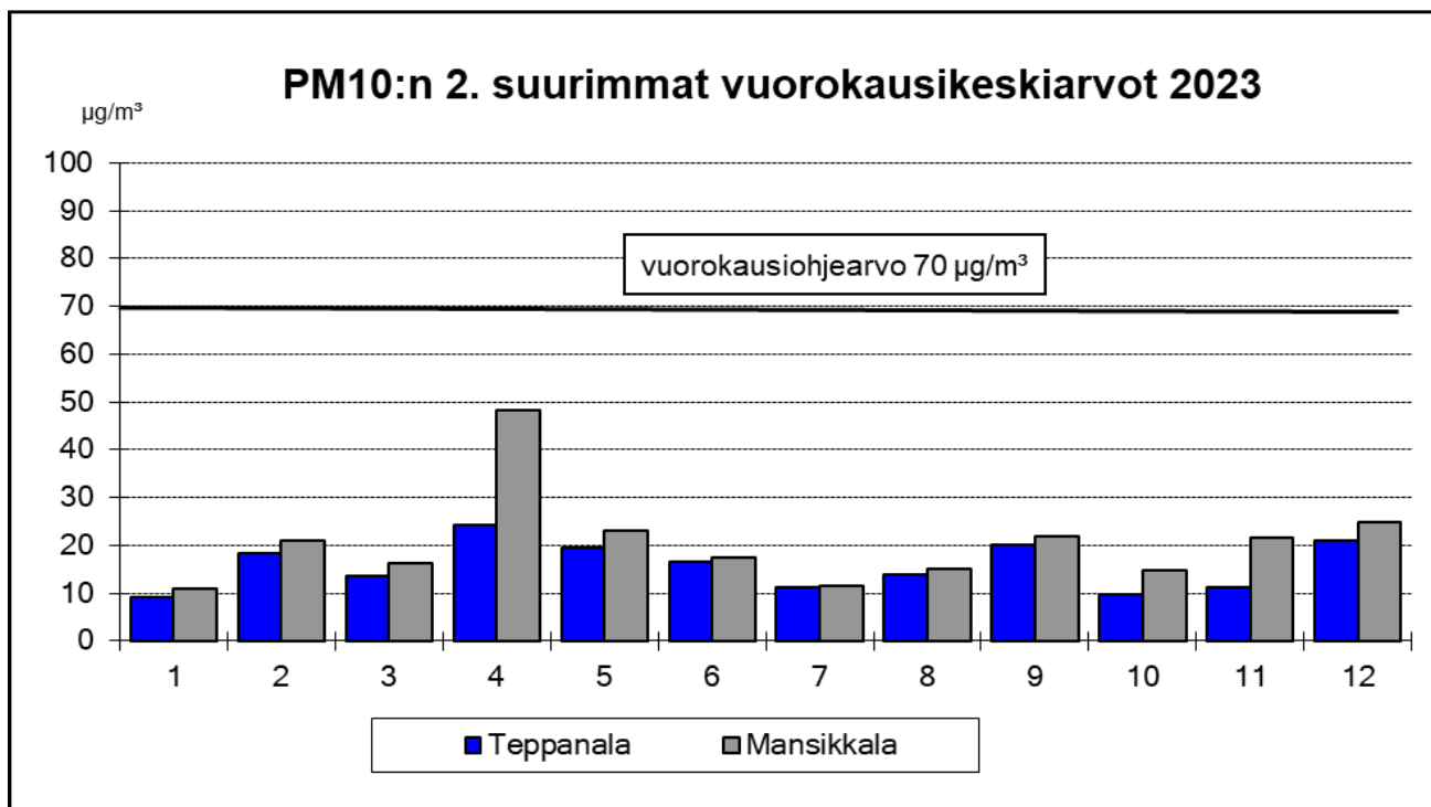
Kuva 25: Mansikkalan ja Teppanalan mittauspisteiden PM10:n kuukausien 2. suurimmat vuorokausikeskiarvot ( \mu\text{g}/\text{m}^3 ) vuonna 2023
