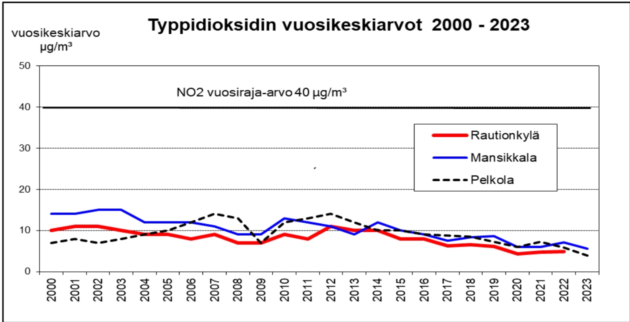
Kuva 23: Imatran Mansikkalan ja Pelkolan typpidioksidin vuosikeskiarvot vuosina 2000–2023, Rautionkylän vuosina 2000 - 2022
