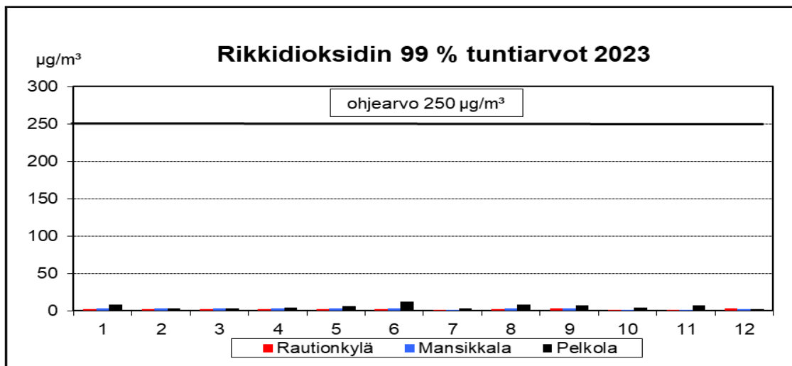
Kuva 15: Imatran mittauspisteiden rikkidioksidin kuukausikeskiarvot (µg/m 3 ) ja tuntiohjearvoon (250 µg/m 3 ) verrattavat pitoisuudet (µg/m 3 ) vuonna 2023
