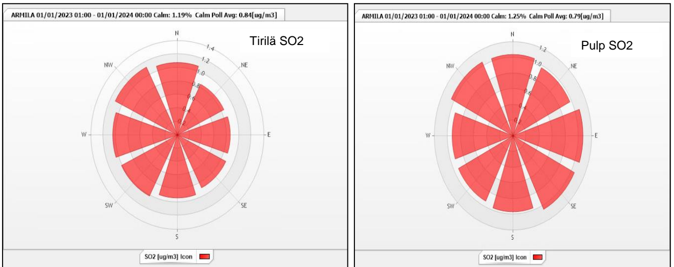
Kuva 40: Tirilän ja Pulpin rikkidioksidin pitoisuuskeskiarvojen tuulensuuntajakaumat sektoreittain vuonna 2023. Armilan sääaseman tuulensuunta, tuulennopeus \geq 0,3 m/s.
