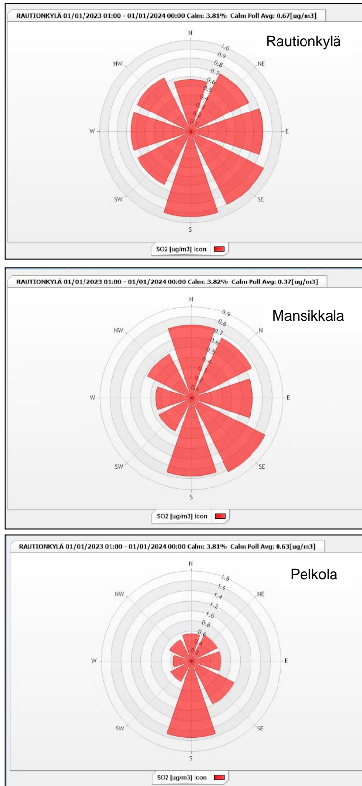
Kuva 17: Imatran Rautionkylän, Mansikkalan ja Pelkolan mittauspisteiden rikkidioksidipitoisuuksien (µg/m 3 ) tuulensuuntajakaumat vuonna 2023. Rautionkylän tuulensuunta, tuulennopeus ≥ 0,3 m/s.
