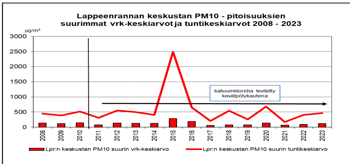
Kuva 51: Lappeenrannan keskustan suurimmat PM10 - vuorokausi- ja tuntikeskiarvot (µg/m³) vuosina 2008 – 2023
