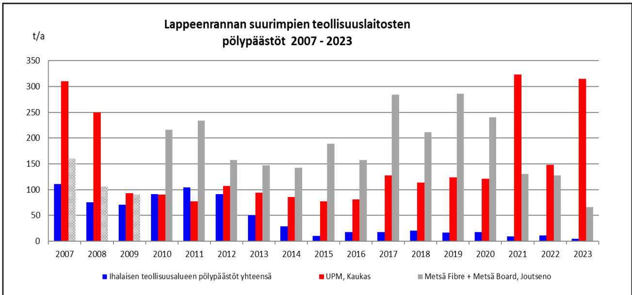
Kuva 5: Ihalaisen teollisuusalueen (Nordkalk Oy Ab ja Finnsementti Oy), UPM Oyj Kaukaan sekä Metsä Fibre Oy Joutsenon tehtaan ja Metsä Board Oyj Joutsenon yhteispölypäästöt (t/a) vuosilta 2007 – 2023 (vain Metsä Fibre Oy Joutsenon tehtaan hiukkaspäästöt vuosilta 2007-2009)
