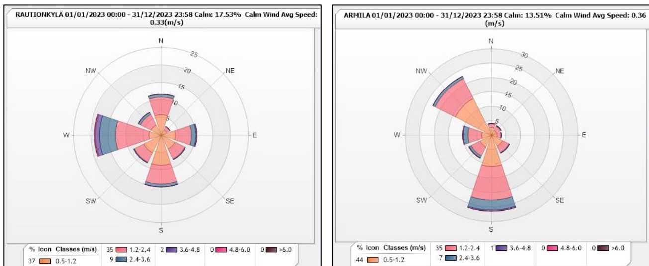
Kuva 8: Imatran Rautionkylän ja Lappeenrannan Armilan sääasemien tuulensuuntajakaumat vuonna 2023
