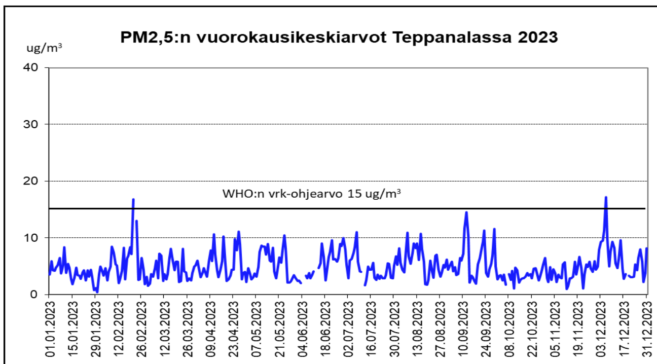
Kuva 26: Imatran Teppanalan PM2,5:n vuorokausikeskiarvot ( \mu\text{g}/\text{m}^3 ) vuonna 2023
