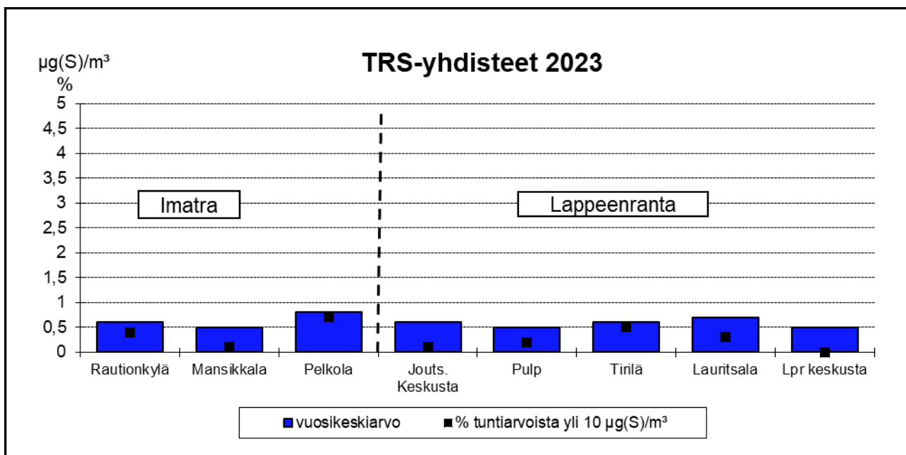
Kuva 59: Imatran ja Lappeenrannan mittauspisteiden vuoden 2023 TRS-yhdisteiden vuosikeskiarvot ja tuntipitoisuuden 10 \mu\text{g(S)}/\text{m}^3 ylitysten %-osuudet
