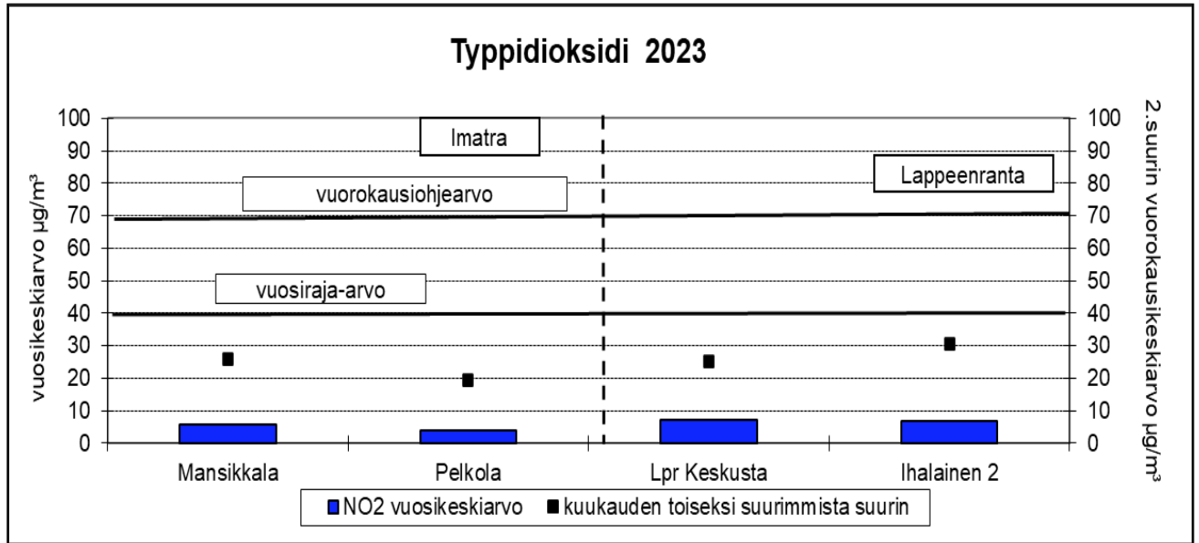
Kuva 66: Imatran ja Lappeenrannan mittauspisteiden typpidioksidin vuosikeskiarvot ja vuorokausiohjeeseen (70 µg/m³) verrattavat pitoisuudet vuonna 2023
