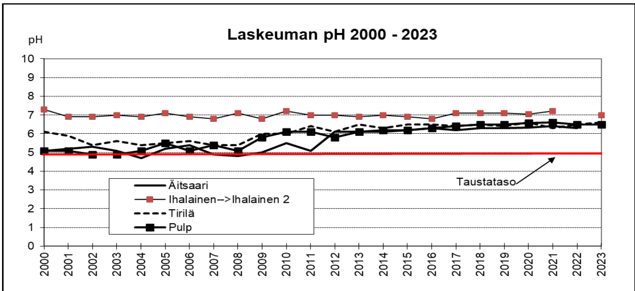
Kuva 56: Lappeenrannan mittauspisteiden rikin, kalsiumin ja pH:n vuosilaskeumat 2000 - 2023. Ihalaisen laskeumapisteen paikkaa muutettiin kesäkuussa 2022, ja uusi piste nimettiin Ihalainen 2:ksi. Äitsaaren laskeuman keräys on lopetettu 31.12.2022
