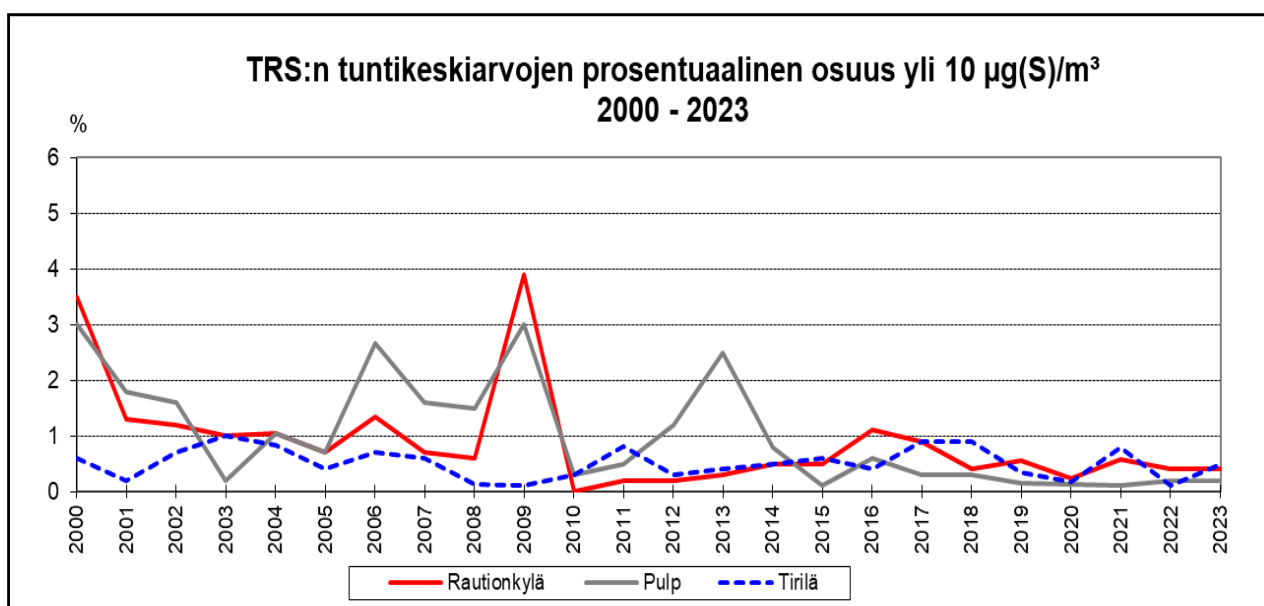
Kuva 60: TRS:n yli 10 \mu\text{g(S)}/\text{m}^3 -tuntikeskiarvopitoisuuksien prosenttiosuudet vuosina 2000 - 2023 Rautionkylässä, Pulpilla ja Tirilässä
