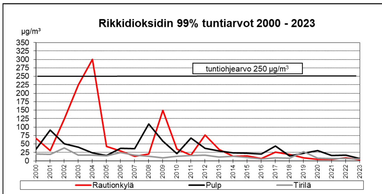
Kuva 62: Rikkidioksidin suurimmat 99% - tuntiarvot vuosina 2000 – 2023
