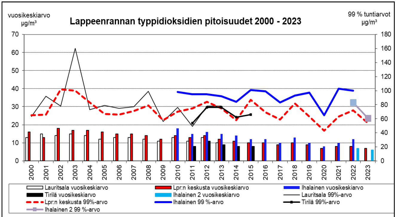
Kuva 45: Lappeenrannan mittauspisteiden NO 2 - vuosikeskiarvot ja 99 %:n suurimmat tunti-arvot vuosina 2000 - 2023 ( \mu\text{g}/\text{m}^3 ). Ihalaisessa mittauksia 1.1. – 30.5.2022 ja Ihalainen 2:ssa 30.7.2022 alkaen
