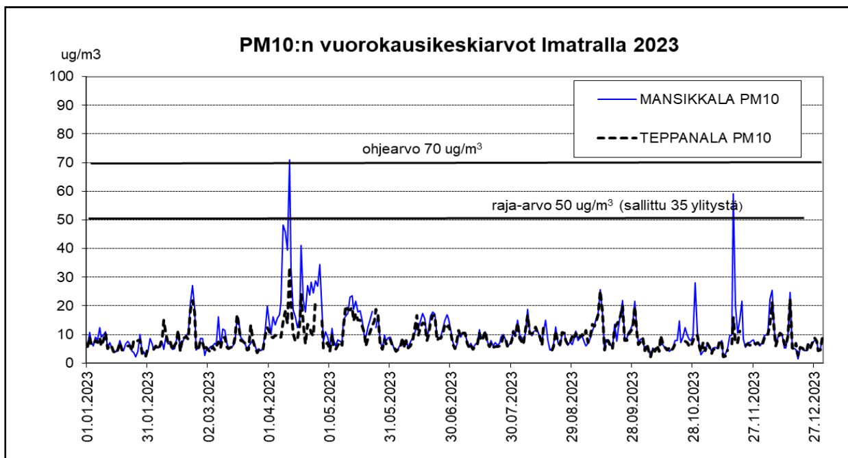
Kuva 24: Imatran Mansikkalan ja Teppanalan mittauspisteiden PM10:n vuorokausikeskiarvot ( \mu\text{g}/\text{m}^3 ) vuonna 2023
