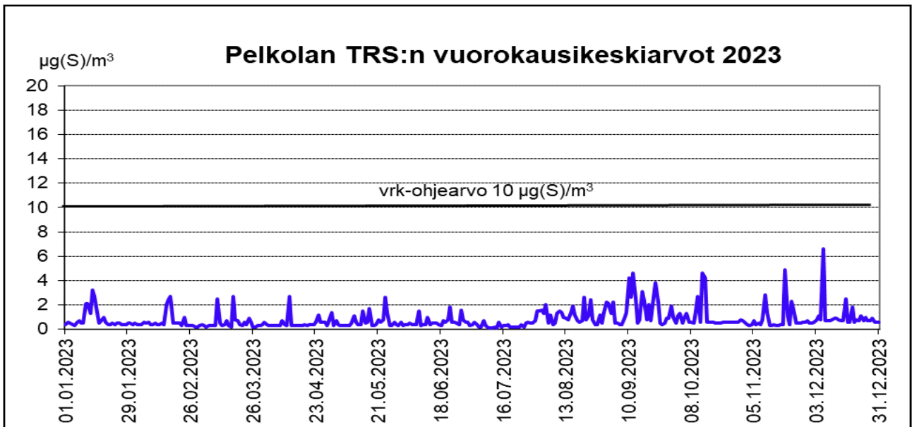
Kuva 11: Rautionkylän, Mansikkalan ja Pelkolan TRS-yhdisteiden vuorokausikeskiarvot ( \mu\text{g(S)}/\text{m}^3 ) vuonna 2023
