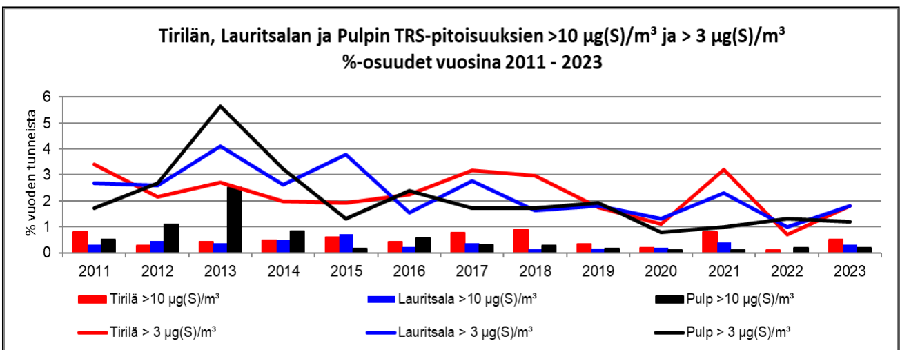
Kuva 37: Tirilän, Lauritsalan ja Pulpin TRS - tuntipitoisuuksien >10 \mu\text{g(S)}/\text{m}^3 ja >3 \mu\text{g(S)}/\text{m}^3 %-osuudet vuosina 2011 – 2023
