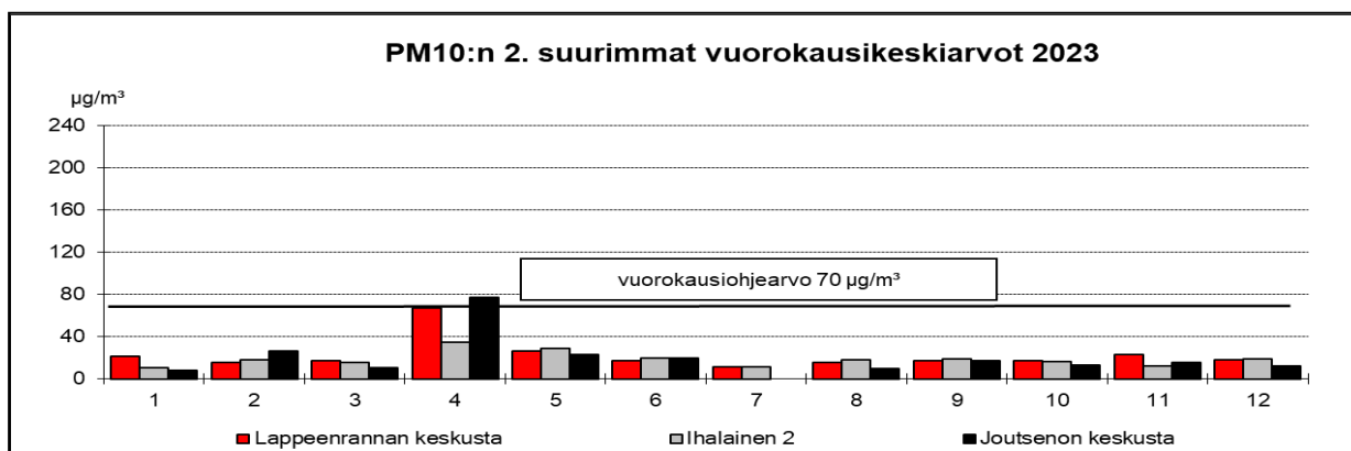
Kuva 46: Lappeenrannan keskustan, Ihalainen 2:n ja Joutsenon keskustan PM10 - kuukausikeskiarvot ja kuukausien 2. suurimmat vuorokausikeskiarvot vuonna 2023 ( \mu\text{g}/\text{m}^3 ).
