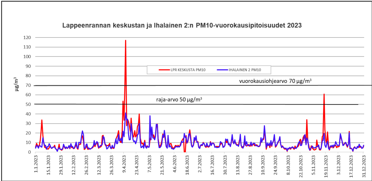
Kuva 47: Lappeenrannan keskustan ja Ihalainen 2:n mittauspisteiden PM10 - vuorokausikeskiarvot ( \mu\text{g}/\text{m}^3 ) vuonna 2023
