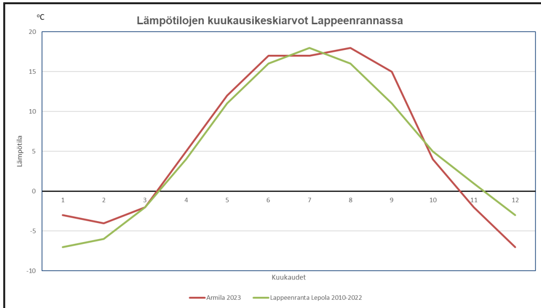
Kuva 9: Armilan sääaseman lämpötilojen kuukausikeskiarvot vuonna 2023 ja Lappeenrannan Lepolan sääaseman (Ilmatieteenlaitos) lämpötilojen kuukausikeskiarvot vuosina 2010 – 2022
