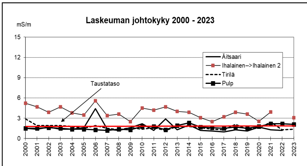
Kuva 57: Lappeenrannan mittauspisteiden laskeuman kokonaisfosforin, kokonaistypen ja johtokyvyn vuosilaskeumat 2000 – 2023. Ihalaisen laskeumapisteen paikkaa muutettiin kesäkuussa 2022, ja uusi piste nimettiin Ihalainen 2:ksi. Äitsaaren laskeuman keräys on lopetettu 31.12.2022
