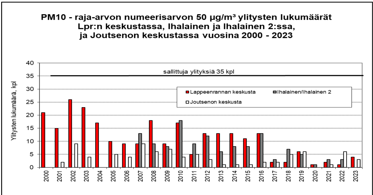
Kuva 48: Lappeenrannan hiukkasmittauspisteiden PM10 - raja-arvon numeerisarvon 50 \mu\text{g}/\text{m}^3 ylitysten lukumäärät 2000 – 2023. Ihalaisen mittauspiste muuttunut Ihalainen 2:ksi 30.5.2022
