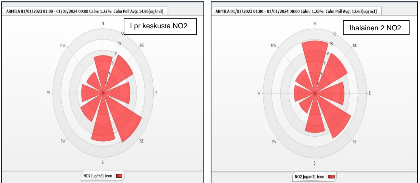
Kuva 43: Lappeenrannan keskustan ja Ihalainen 2:n NO 2 - tuntipitoisuuskeskiarvojen tuulensuuntajakaumat sektoreittain vuonna 2023. Armilan tuulensuunta, tuulennopeus ≥ 0,3 m/s
