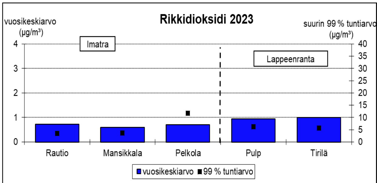
Kuva 61: Imatran ja Lappeenrannan mittauspisteiden vuoden 2023 rikkidioksidin vuosikeskiarvot ja tuntiohjeeseen verrattavat pitoisuudet (suurimmat kuukausien 99 % -tuntiarvoista).
