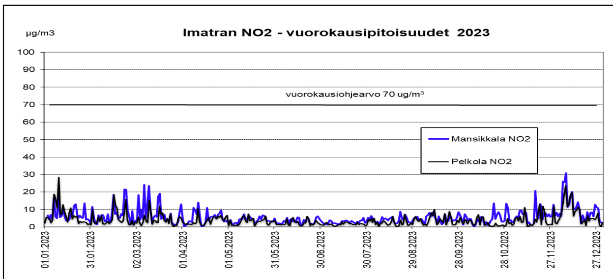
Kuva 20: Imatran mittauspisteiden NO 2 - vuorokausikeskiarvot (µg/m 3 ) vuonna 2023
