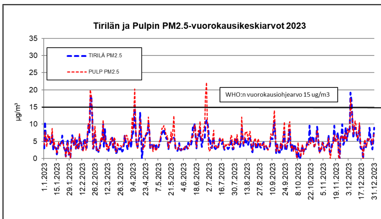
Kuva 53: Tirilän ja Pulpin PM2,5 - vuorokausikeskiarvot vuonna 2023 ( \mu\text{g}/\text{m}^3 )
