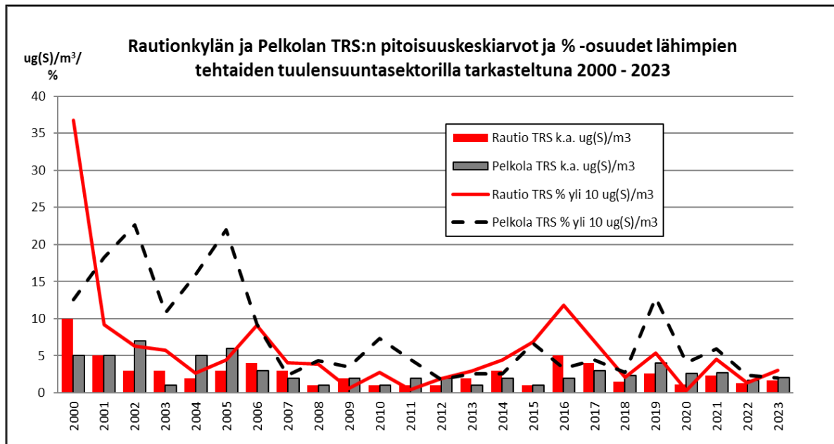
Kuva 14b: Rautionkylän ja Pelkolan TRS-vuosikeskiarvot ja prosenttiosuudet lähimmän tehtaan tuulensuuntasektorilla tarkasteltuna (Rautionkylässä Stora Enson Kaukopään tuulensuunnalla ja Pelkolassa Svetogorskin tehtaiden tuulensuunnalla) vuosina 2000–2023 (arvot taulukosta 13)
