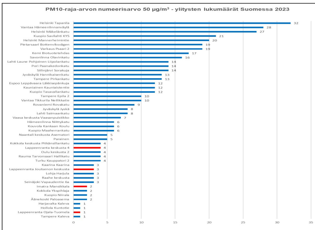
Kuva 52: Etelä-Karjalan PM10 - mittauspisteiden yli 50 µg/m³ vuorokausikeskiarvojen määrä verrattuna Suomen muiden PM10- mittauspisteiden vastaaviin lukuihin vuonna 2023. Lähteenä Ilmatieteen laitoksen ilmanlaatuportaalin tarkistamattomat mittaustulokset.
