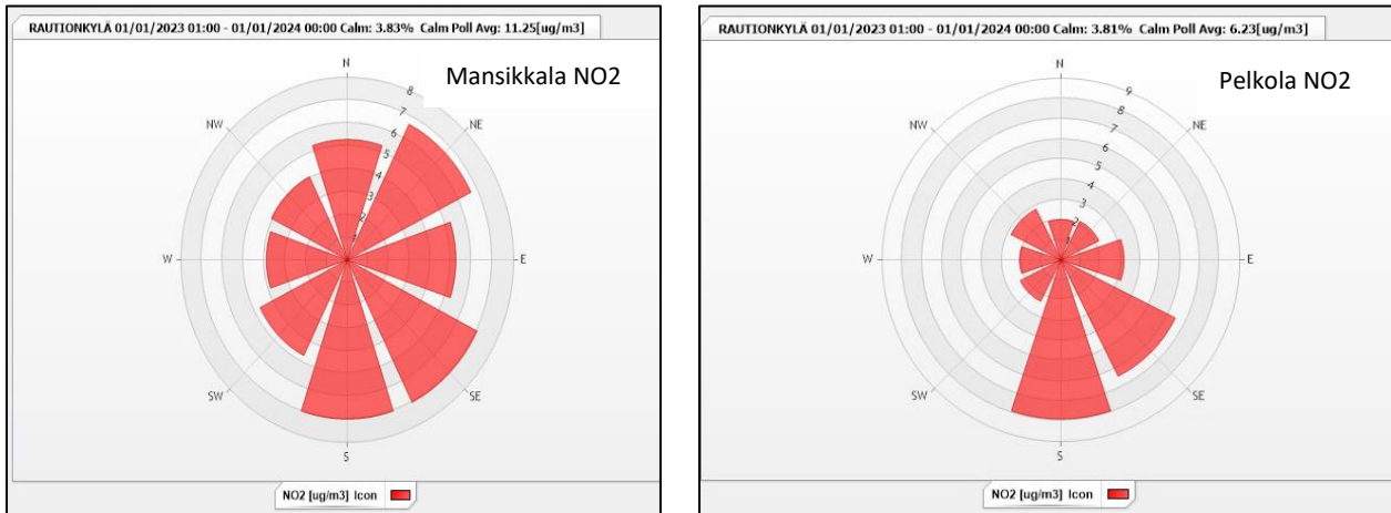
Kuva 22: Imatran Mansikkalan ja Pelkolan mittauspisteiden typpidioksidipitoisuuksien ( \mu\text{g}/\text{m}^3 ) tuulensuuntajakaumat vuonna 2023. Rautionkylän tuulensuunta, tuulennopeus \geq 0,3 m/s.
